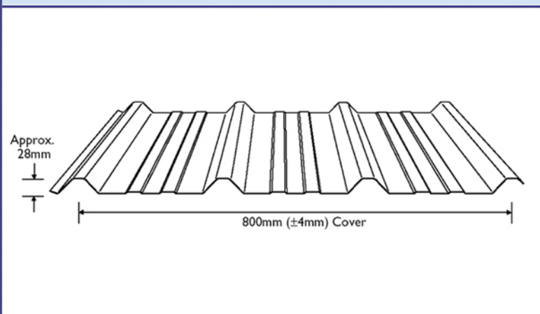
Stramit Mega Clad
