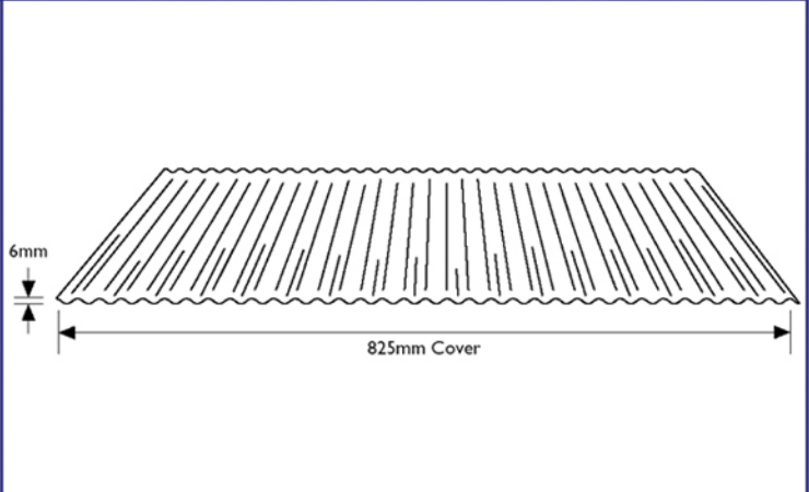
Stramit Mini Rib
