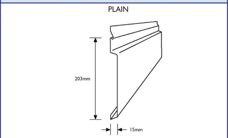
Stramit C Clad
